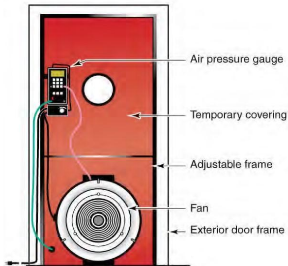
Blower Door Assembly
